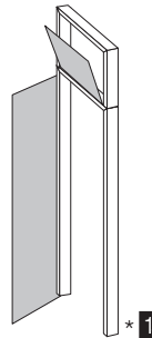
13. Porta con sopra luce apribile a wasistas Door with pull-up opening transom
